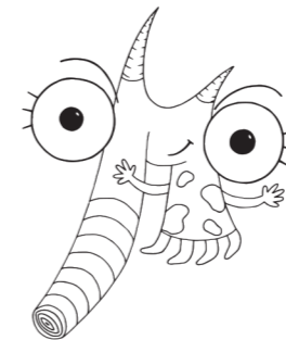
Muon
