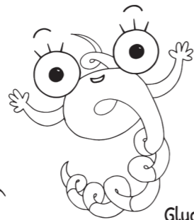
Gluon
